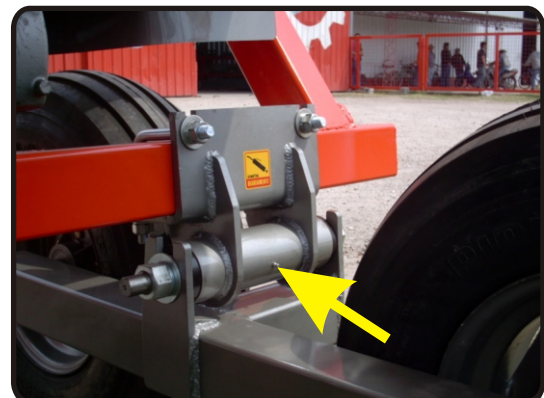
Eje pivot tren rodante
